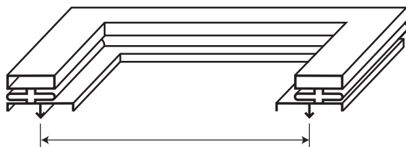
Profil à clipser Donnez les dimensions d'axe en axe
